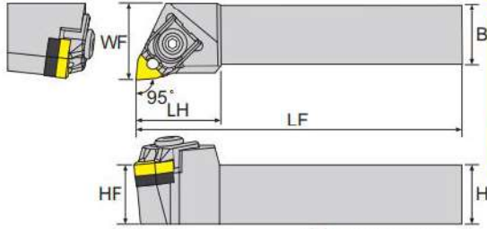
寸法 Dimension(mm)
