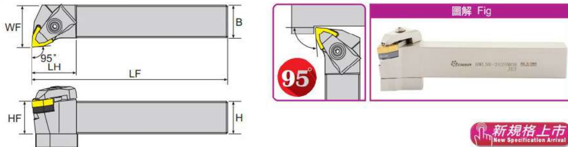
寸法 Dimension(mm)
