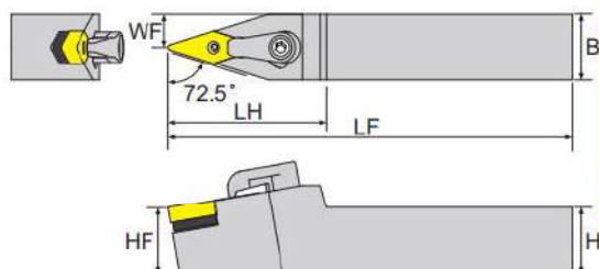
寸法 Dimension(mm)
