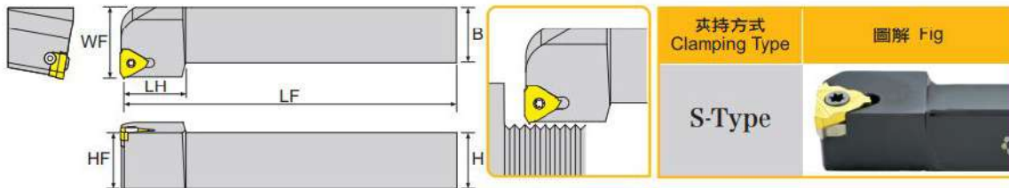
寸法 Dimension(mm)
