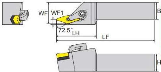
寸法 Dimension(mm)
