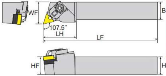
寸法 Dimension(mm)
