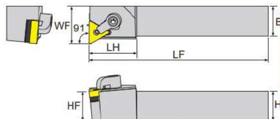
寸法 Dimension(mm)
