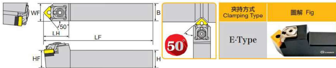
寸法 Dimension(mm)
