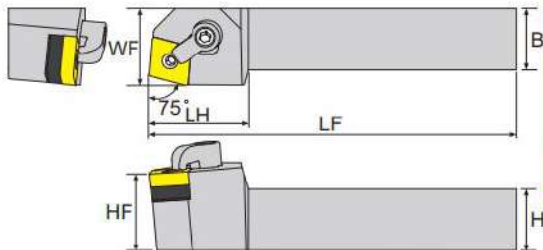
寸法 Dimension(mm)
