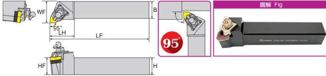
寸法 Dimension(mm)
