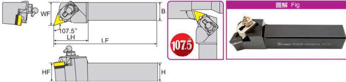
寸法 Dimension(mm)
