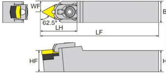
寸法 Dimension(mm)
