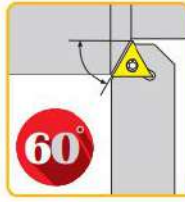
寸法 Dimension(mm)
