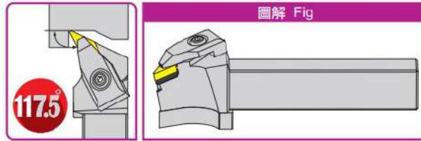
寸法 Dimension(mm)
