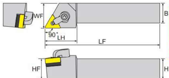
寸法 Dimension(mm)
