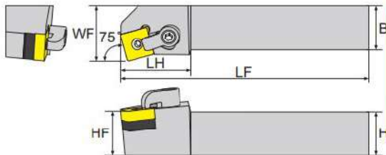
寸法 Dimension(mm)
