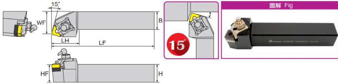
寸法 Dimension(mm)
