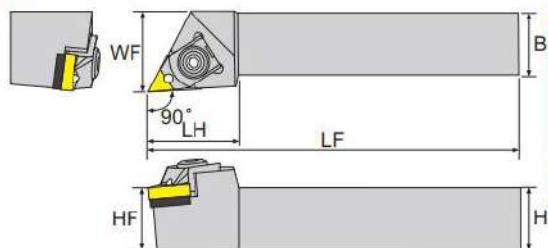
寸法 Dimension(mm)
