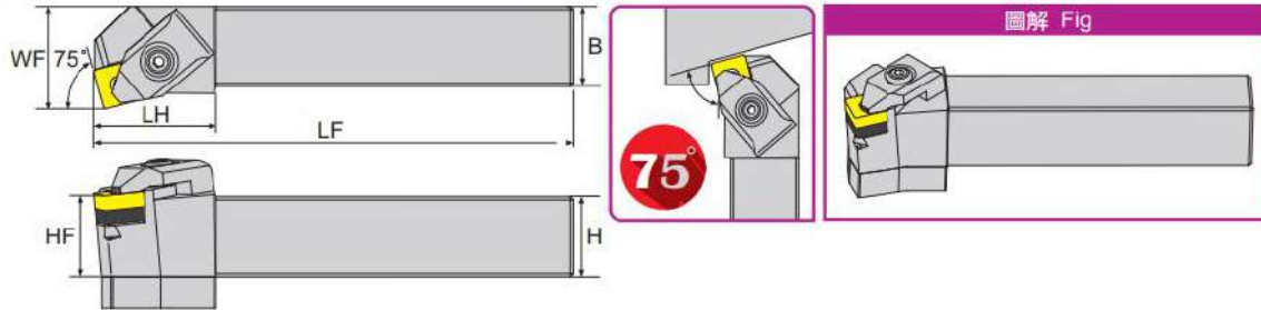
寸法 Dimension(mm)
