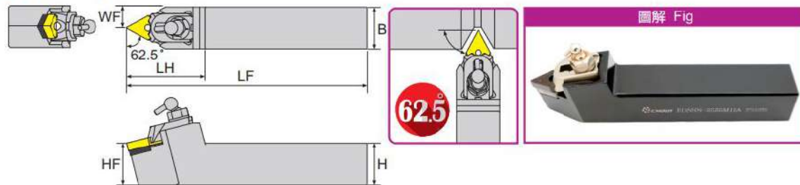
寸法 Dimension(mm)
