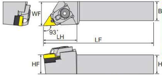
寸法 Dimension(mm)
