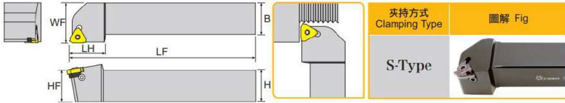
寸法 Dimension(mm)
