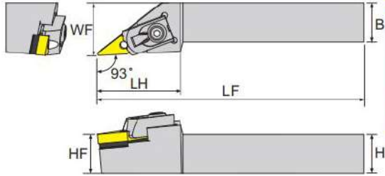
寸法 Dimension(mm)
