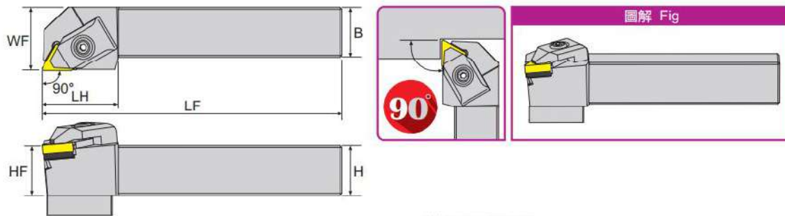
寸法 Dimension(mm)
