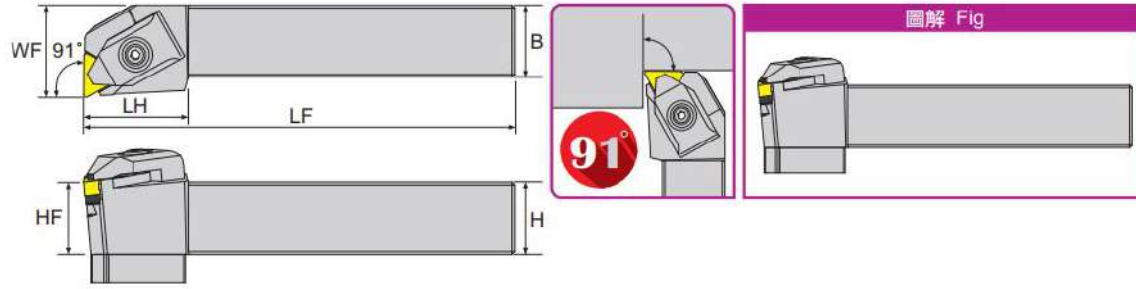
寸法 Dimension(mm)
