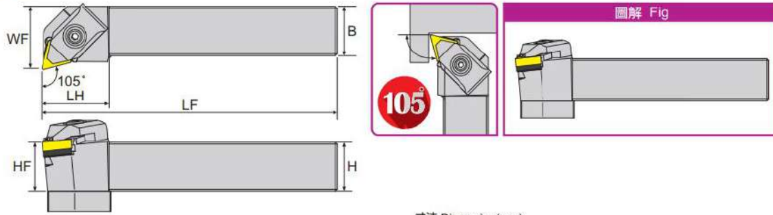
寸法 Dimension(mm)
