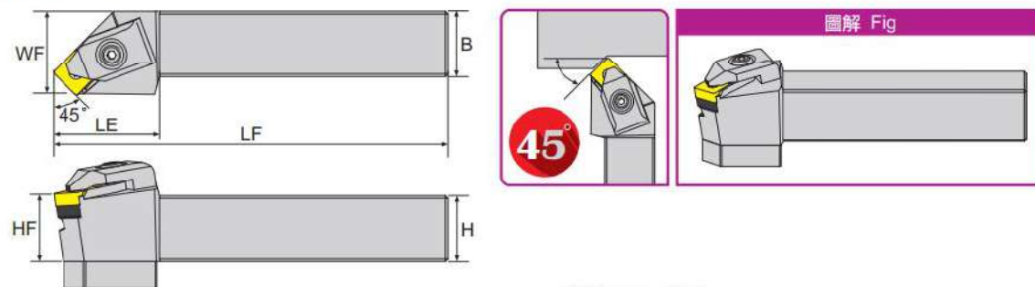
寸法 Dimension(mm)
