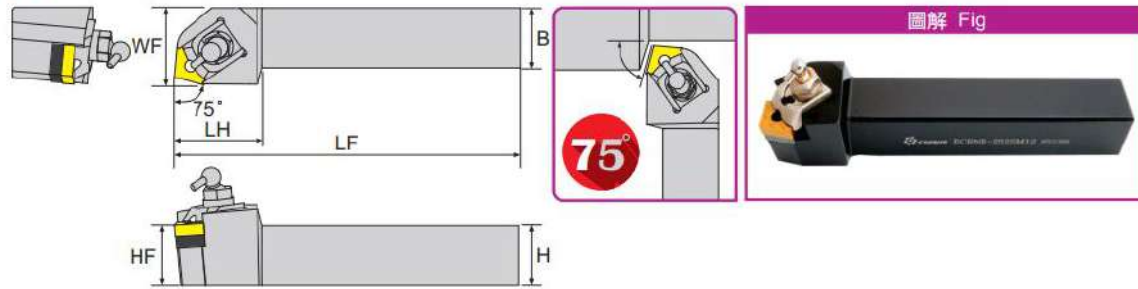
寸法 Dimension(mm)
