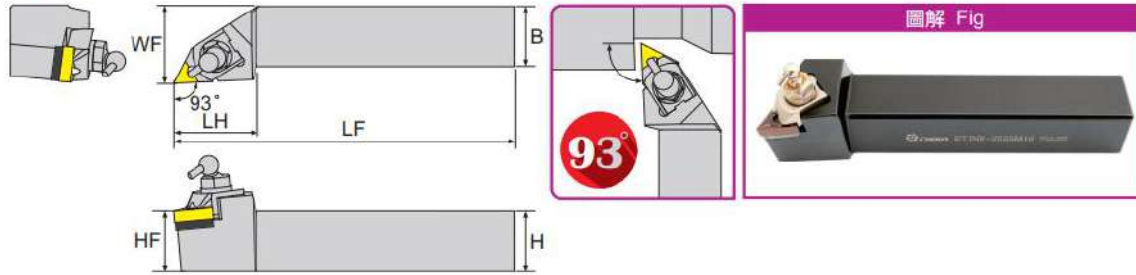
寸法 Dimension(mm)
