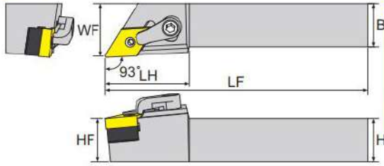
寸法 Dimension(mm)
