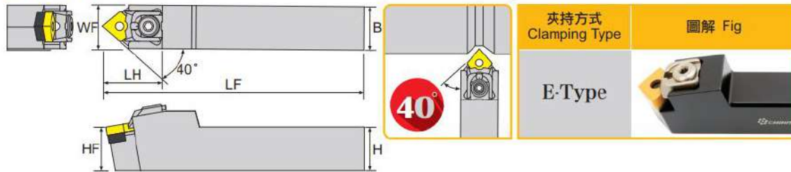
寸法 Dimension(mm)
