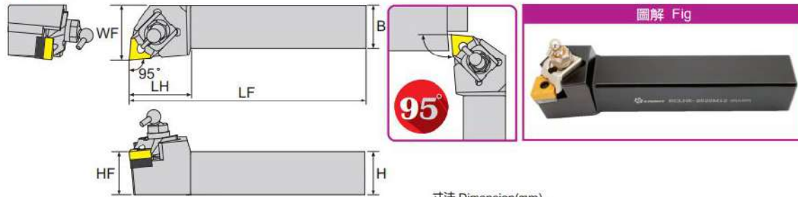
寸法 Dimension(mm)
