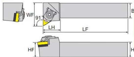
寸法 Dimension(mm)
