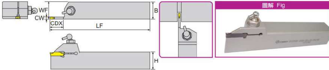
寸法 Dimension(mm)
