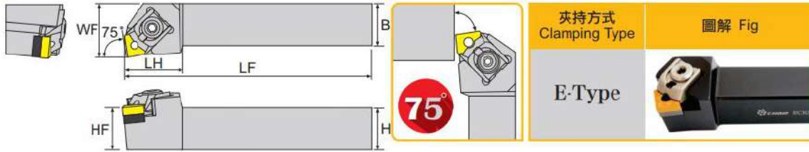
寸法 Dimension(mm)
