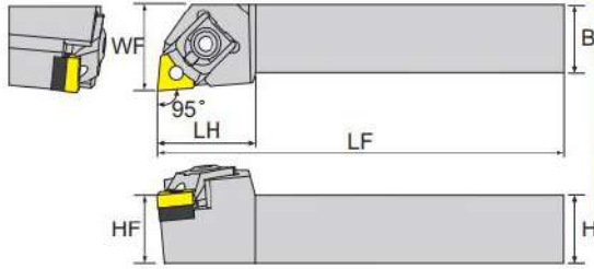
寸法 Dimension(mm)
