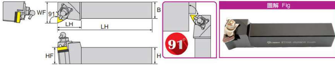
寸法 Dimension(mm)
