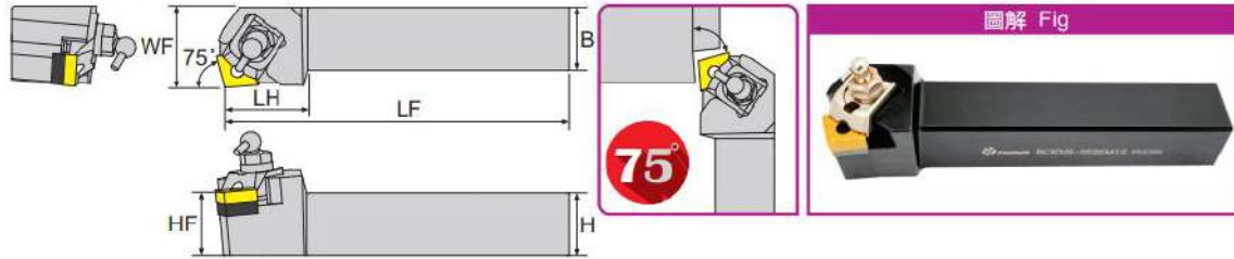
寸法 Dimension(mm)
