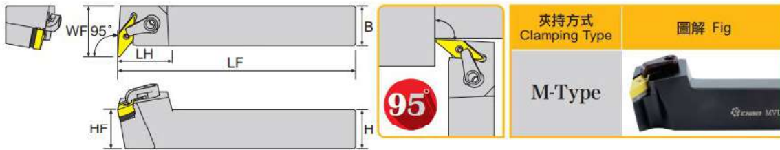
寸法 Dimension(mm)
