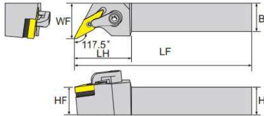
寸法 Dimension(mm)
