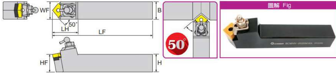
寸法 Dimension(mm)
